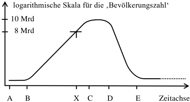
Abbildung 1: Eine Bakterien-Kultur auf einer begrenzten Nahrungsmenge 328 (schematisch)
